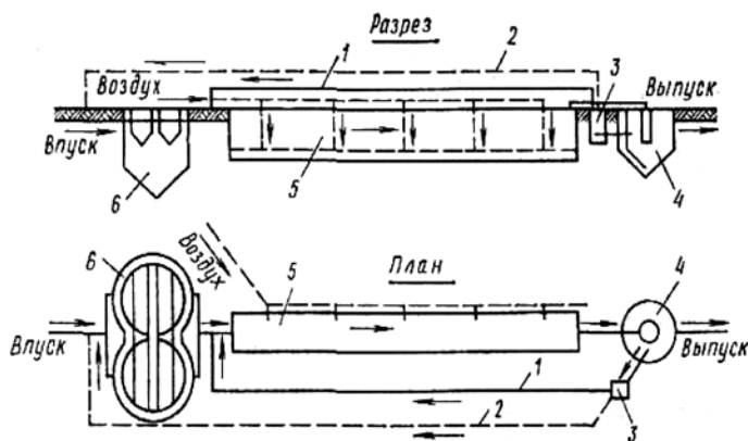
1 – циркулирующий активный ил; 2 – избыточный активный ил; 3 – насосная станция; 4 – вторичный отстойник; 5 – аэротенк; 6 – первичный отстойник
